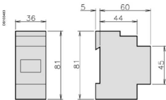
iEM2100/iEM2105 dimensions
