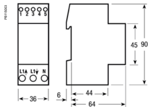
iEM2110/iEM2135/iEM2150/iEM2155 dimensions
